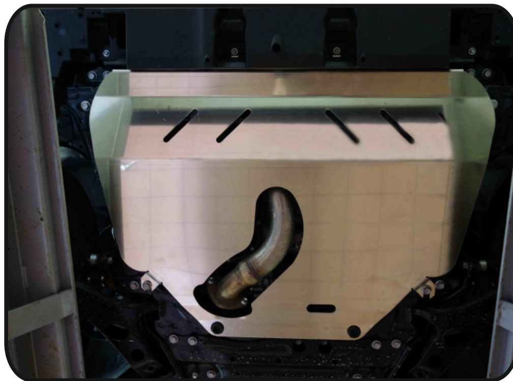
Защита картера (алюминий) 4мм арт.ZKTCC00115
