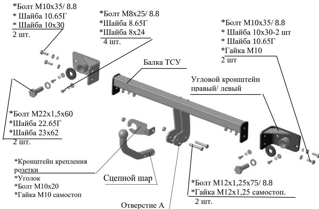
Рис.1 Тягово-сцепное устройство ТСУ 2182.
