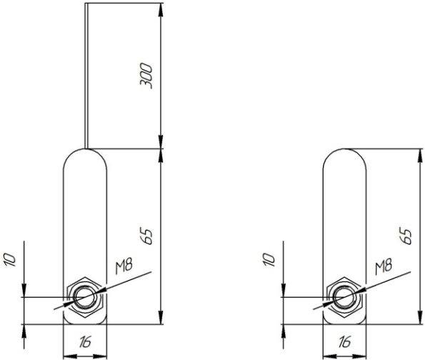
Схема установки
