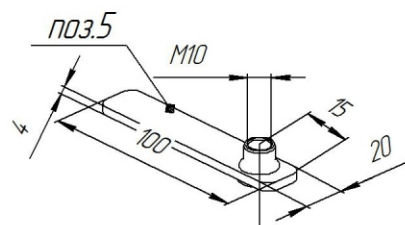
Закладной кронштейн М10 (поз.5)
