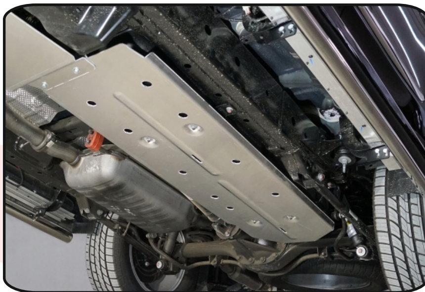
Защита бака (алюминий) 4мм арт. ZKTCC00407.
