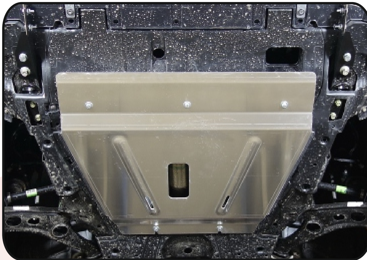
Защита картера и КПП (алюминий) 4 мм арт. ZKTCC00341.
