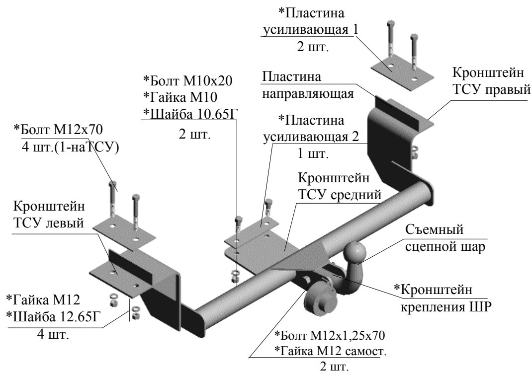
Рис.1 Тягово-сцепное устройство ТСУ 2112.C
