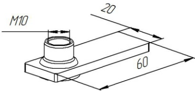
Закладной кронштейн M10 60x20 (поз 4)
