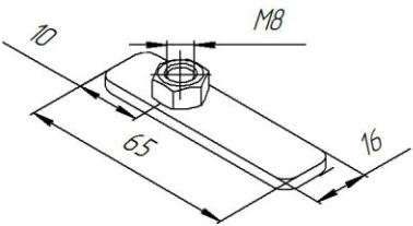
Закладной кронштейн (z-47 M8)
