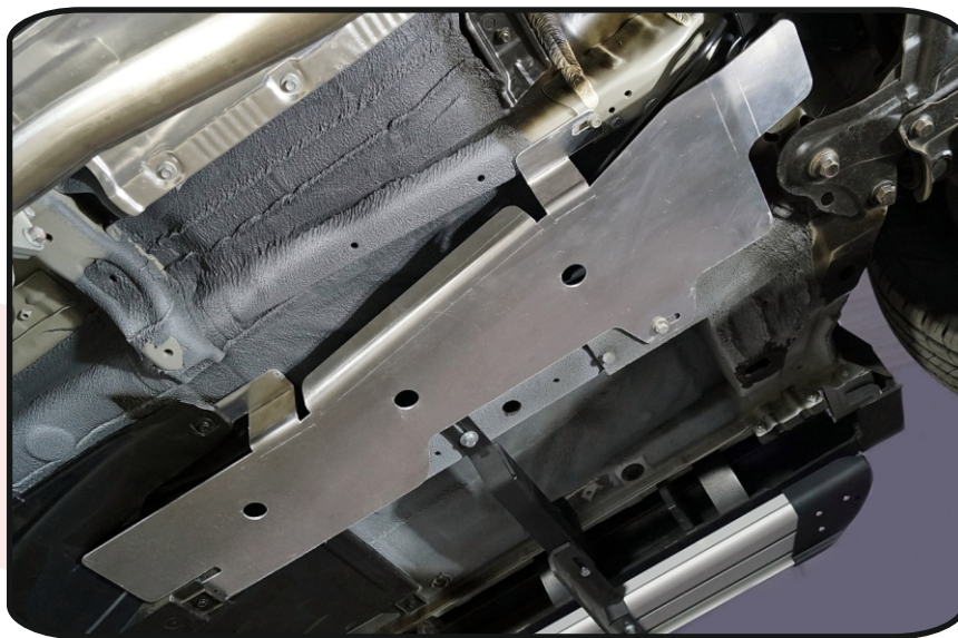
Защита топливopовода (алюминий) 4мм арт. ZKTCC00604
