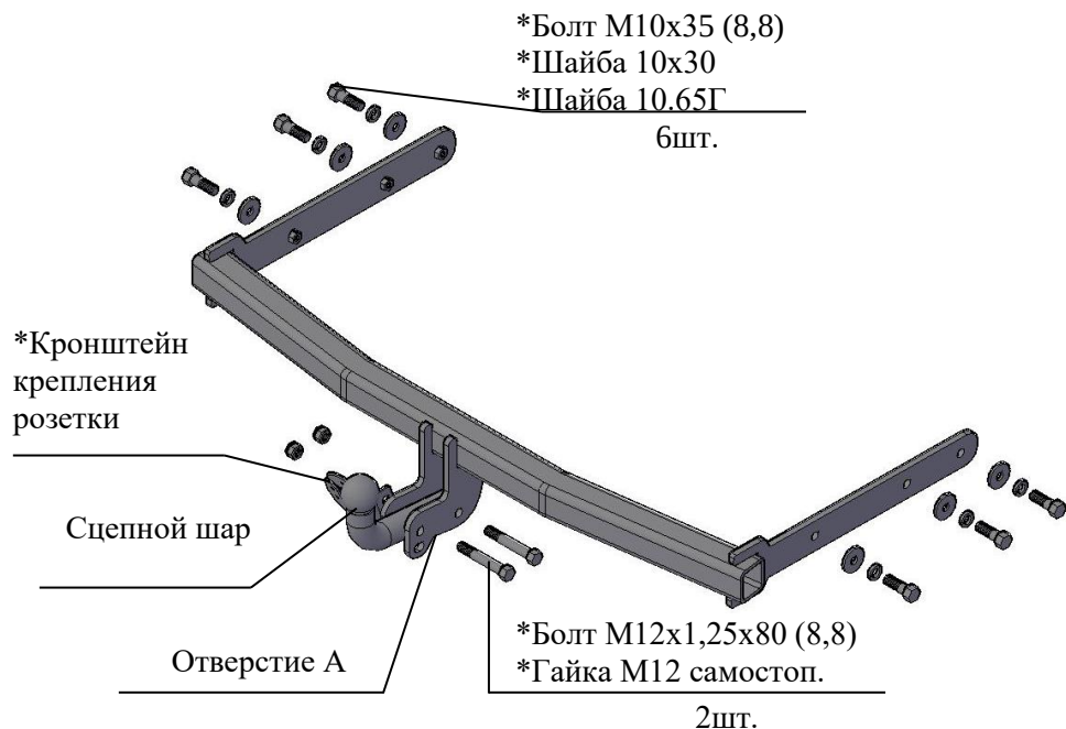
Рис.1 Тягово-сцепное устройство ТСУ 9730
