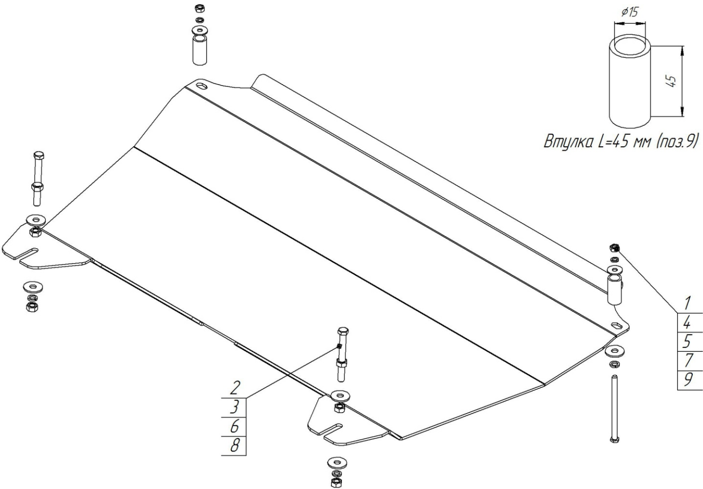
Схема установки
