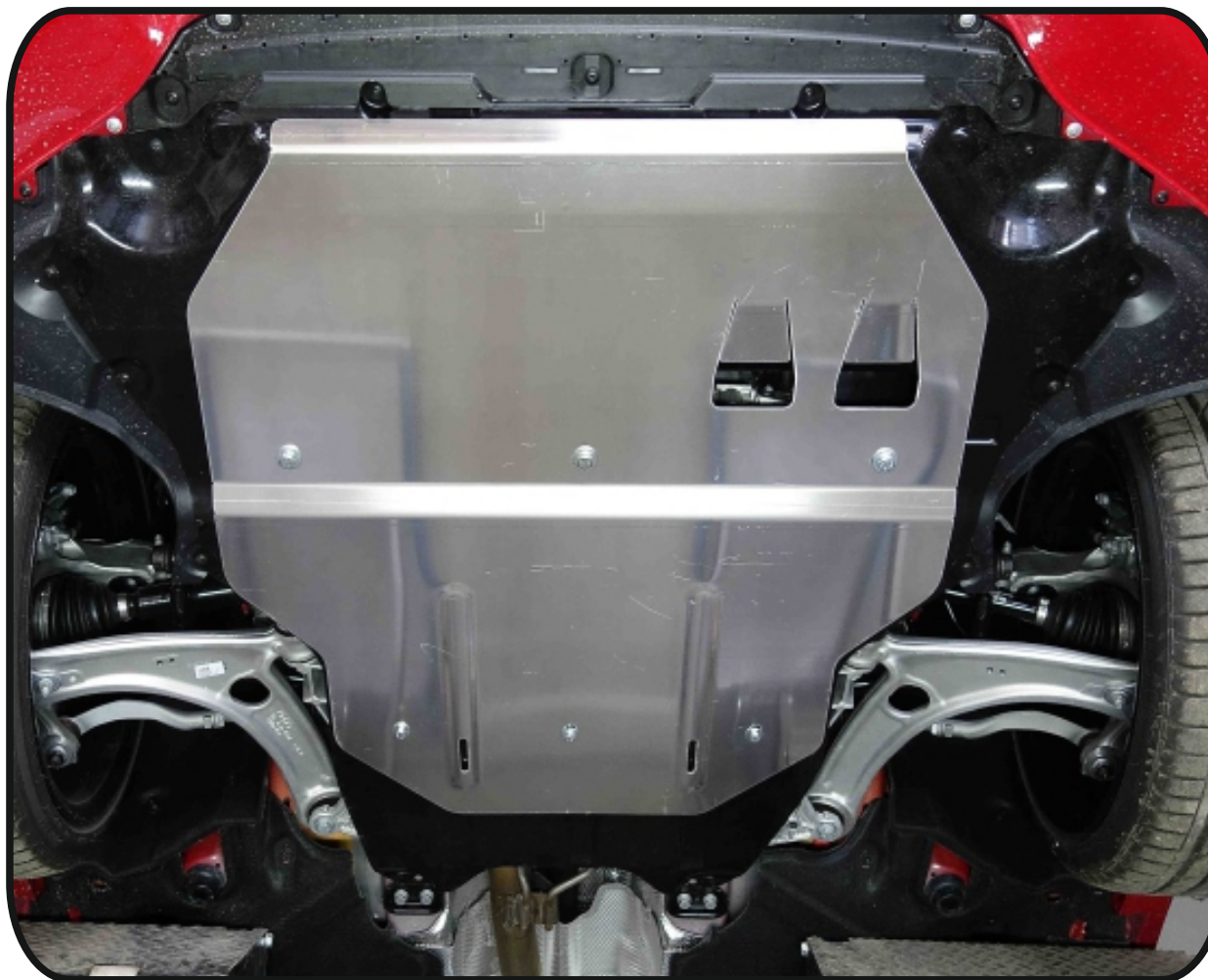
Защита картера (алюминий) 4мм арт.ZKTCC00202
