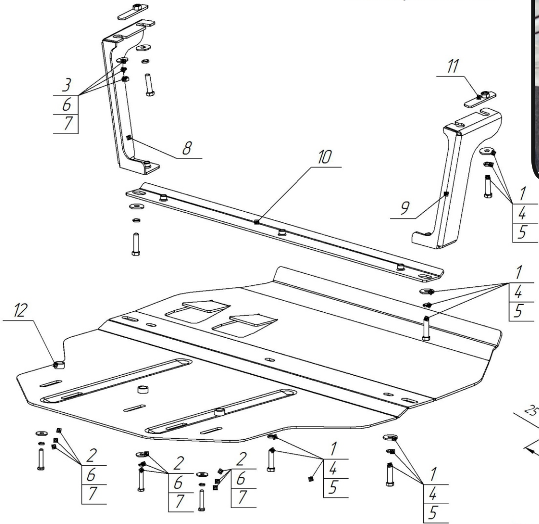
Схема установки
