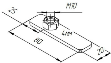
Закладной кронштейн (поз.11)
