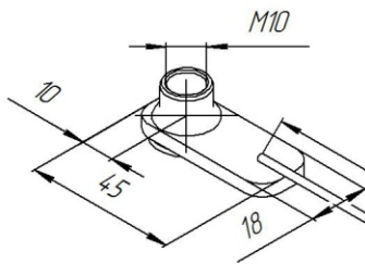
Закладной кронштейн M10 (поз.4)
