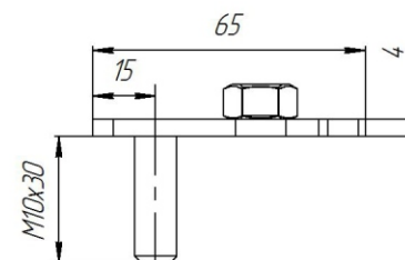
Закладной кронштейн M10 (поз.8)
