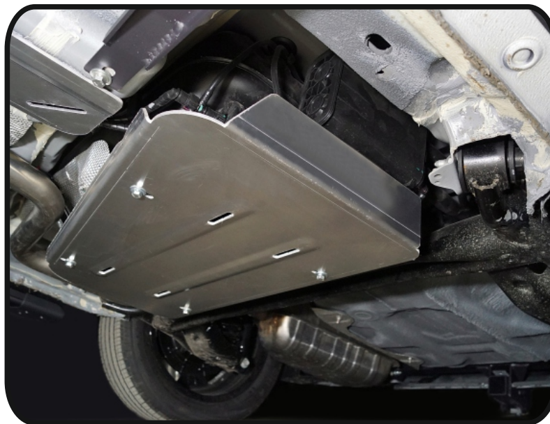
Защита бака и адсорбера (алюминий) 4 мм арт.ZKTCC00567
