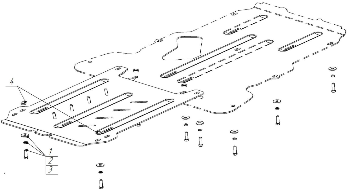
Схема установки
