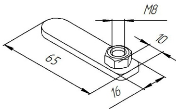
Закладной кронштейн с гайкой (поз.5)
