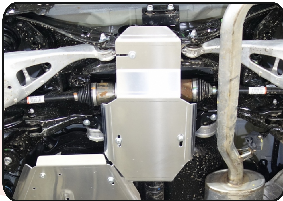
Защита дифференциала (алюминий) 4мм арт. ZKTCC00343.
