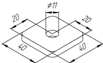
Планка 40x40 S=6 мм
