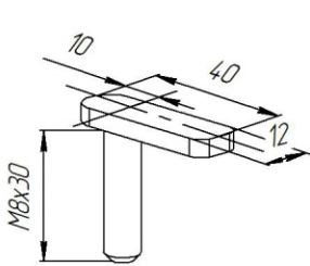
Кронштейн закладной M8x30 (поз.5)
