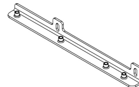
Кронштейн передний (поз.4)
