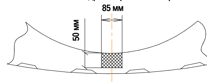
Эскиз подрезки кромки бампера
