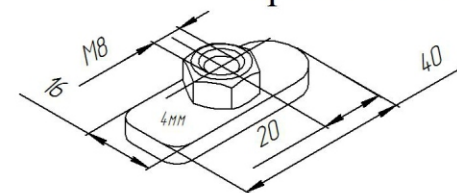
Закладной кронштейн М8 40х16 (поз.9)
