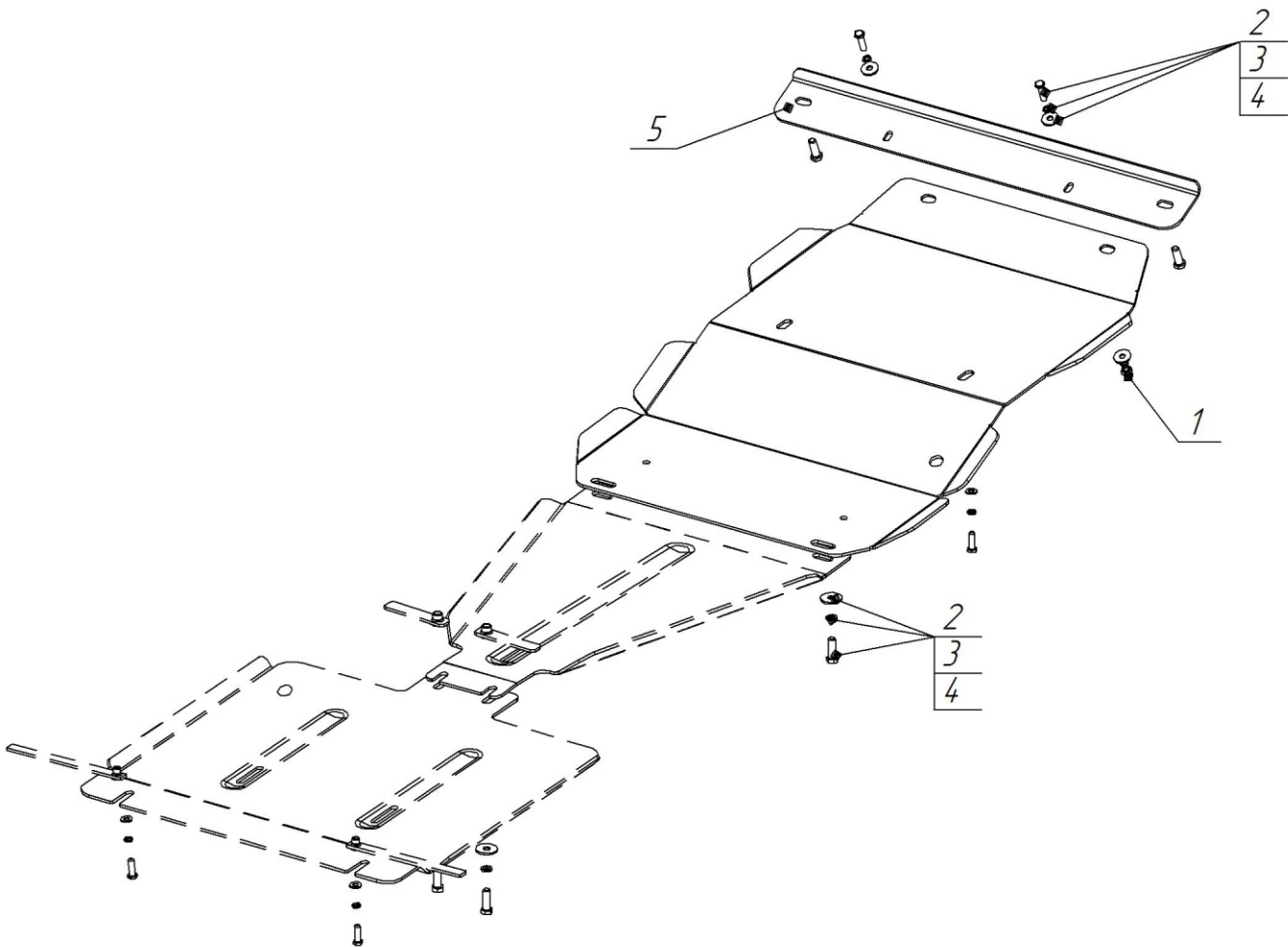
Схема установки
