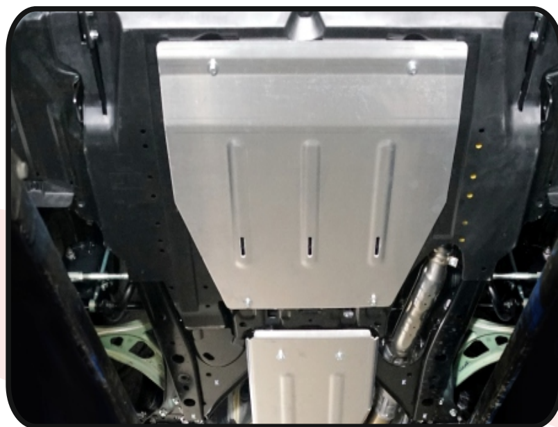
Защита картера (алюминий) 4 мм арт. ZKTCC00511.
