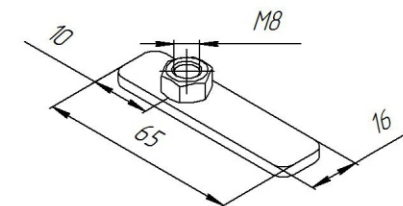
Закладной кронштейн (z-47 M8)
