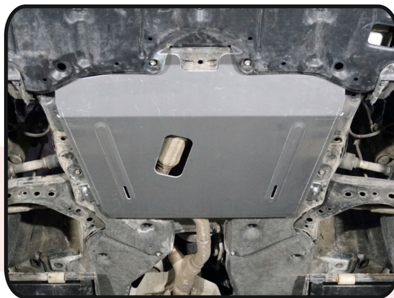
Защита картера и кпп (алюминий) 4 мм арт. ZKTCC00472.
