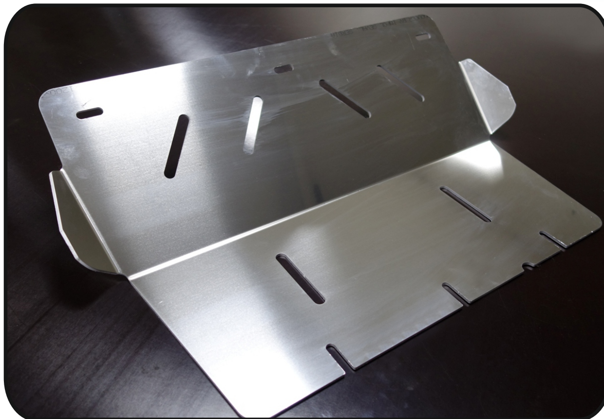
Защита картера (алюминий) 4мм арт.ZKTCC00100 (Не устанавливается без ZKTCC00101)
