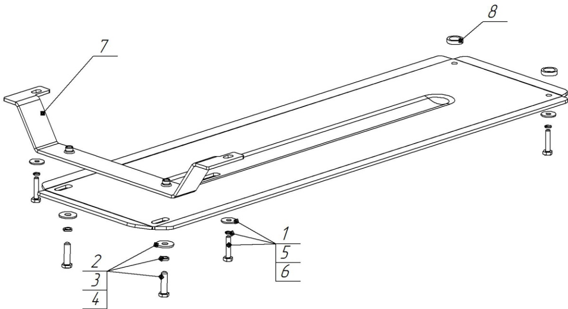
Схема установки
