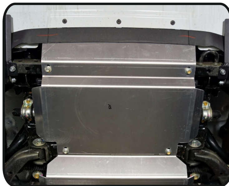
Защита радиаторов (алюминий) 4 мм арт.ZKTCC00521.
