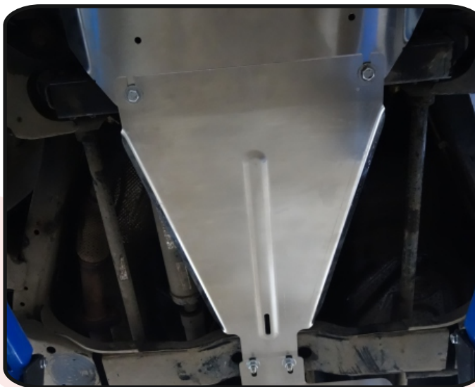
Защита КПП (алюминий) 4мм арт.ZKTCC00088
