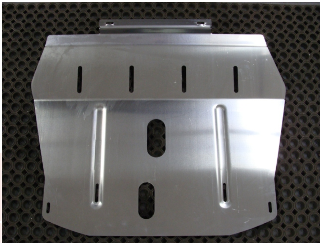
Защита картера (алюминий) 4 мм арт. ZKTCC00064
