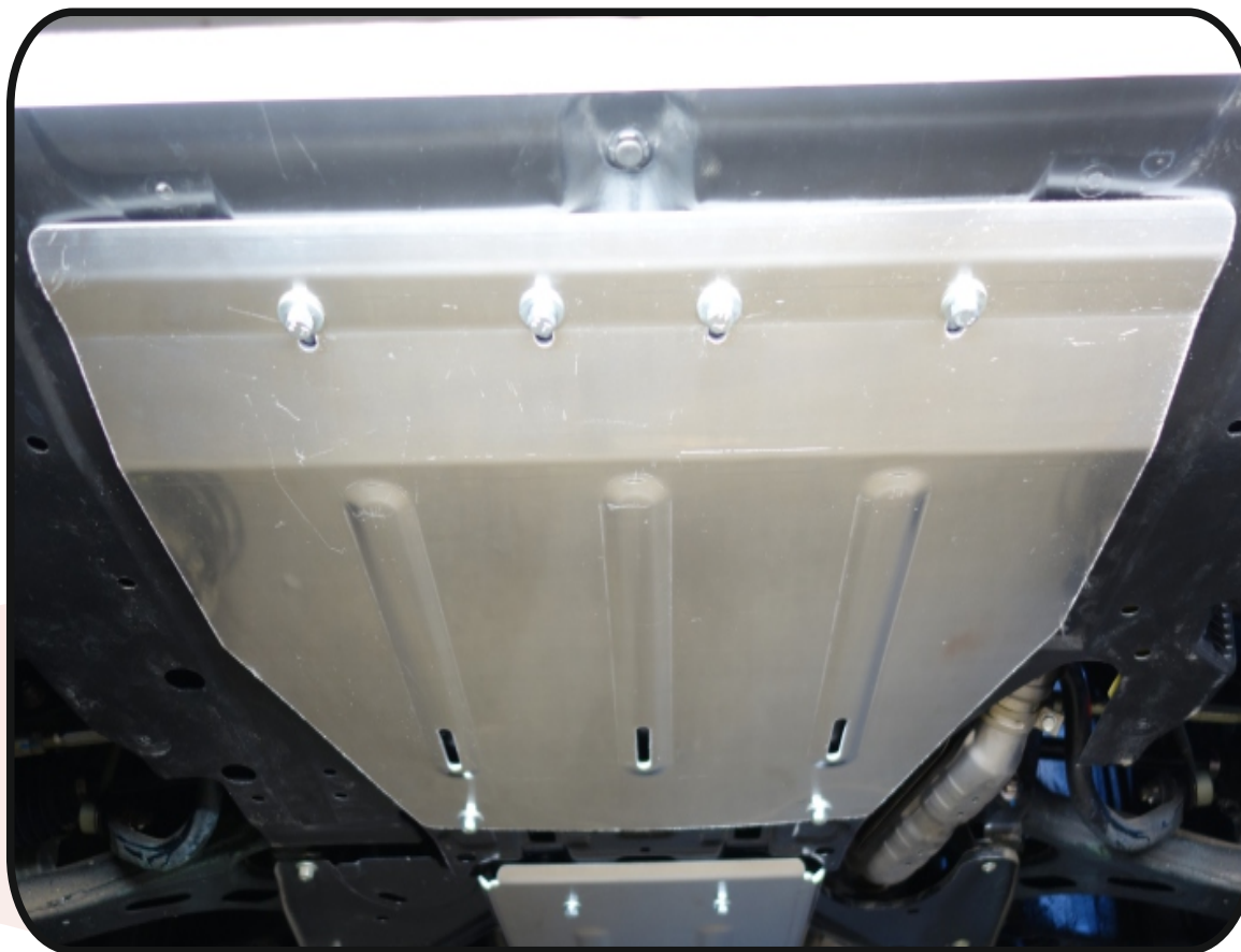
Защита картера (алюминий) 4 мм арт. ZKTCC00320.
