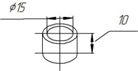
Втулка (поз.8)
