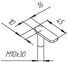
Закладной кронштейн M10x30 (поз.7)
