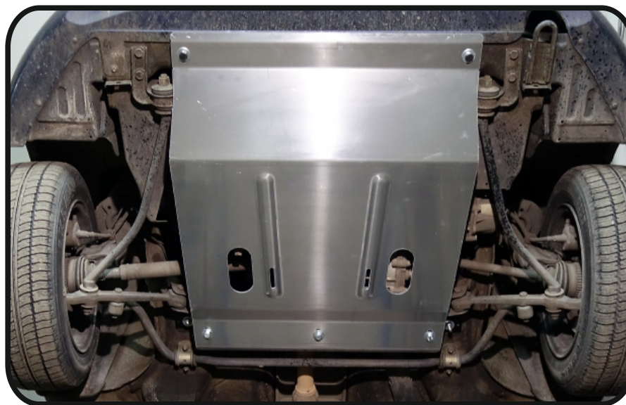
Защита картера (алюминий) 4мм арт.ZKTCC00138
