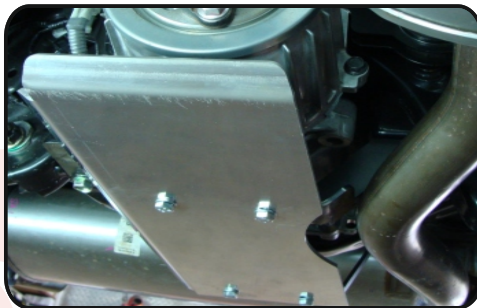
Защита дифференциала (алюминий) 4 мм арт. ZKTCC00068
