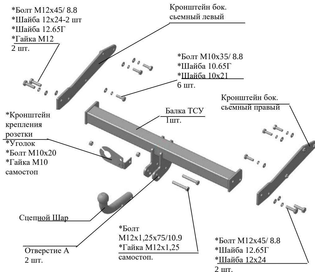
Рис.1 Тягово-сцепное устройство 9180
