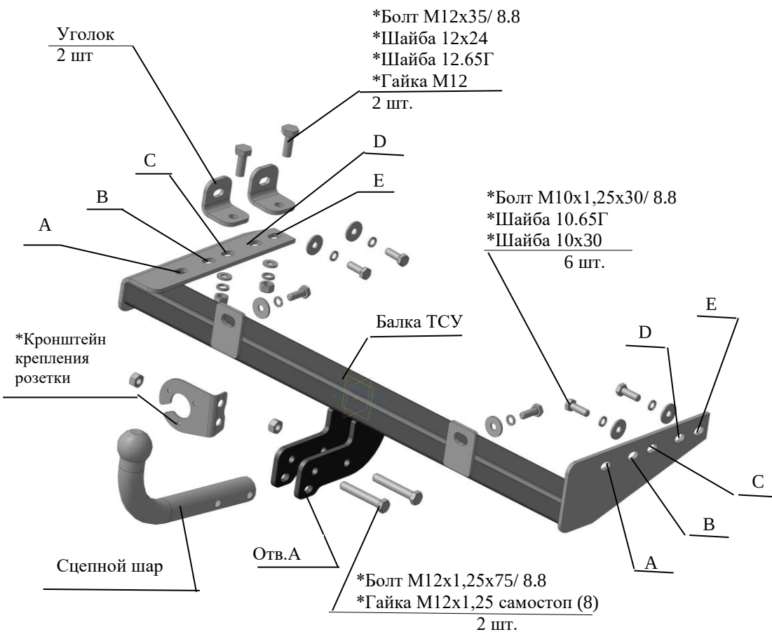
Рис.1 Тягово-сцепное устройство ТСУ 2194.
