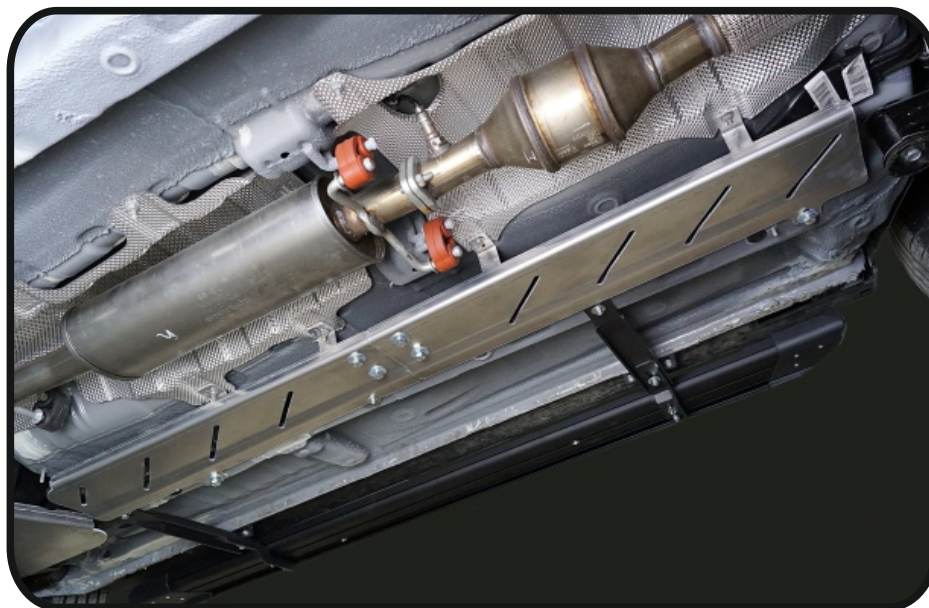
Защита топливопровода (алюминий) 4 мм (комп 2шт) арт.ZKTCC00568
