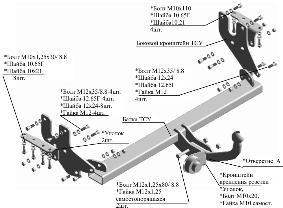
Рис.1 Тягово-сцепное устройство 7130
