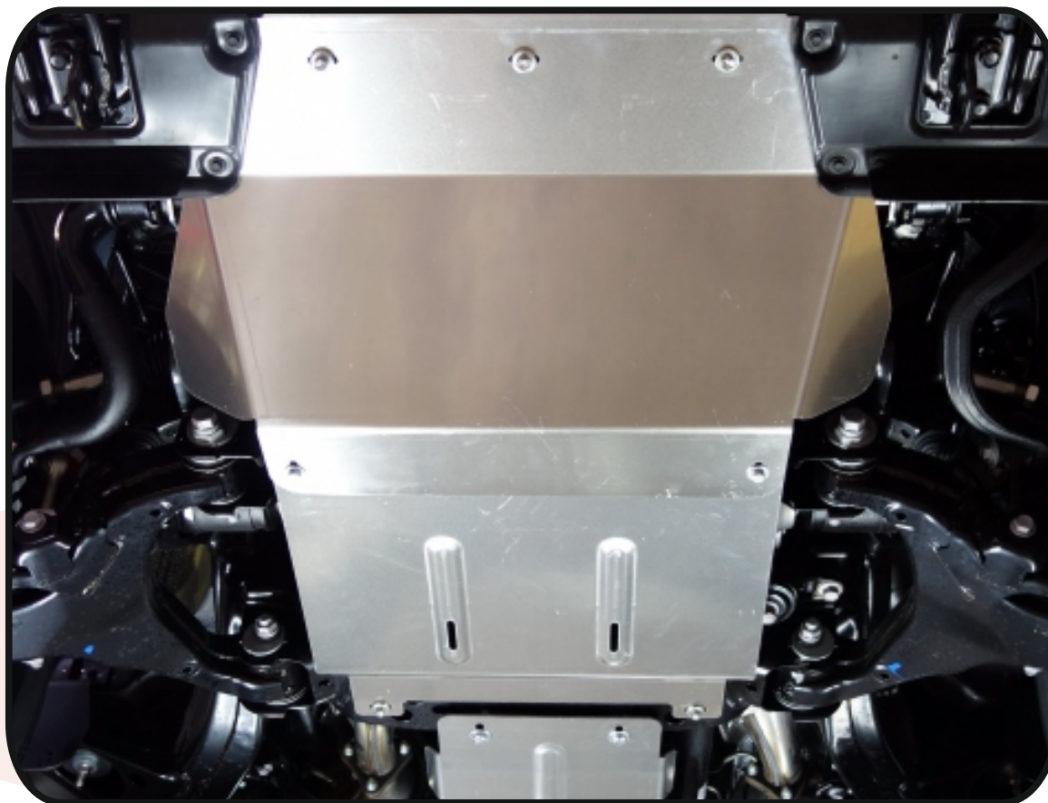
Защита картера (алюминий) 4 мм арт. ZKTCC00035
