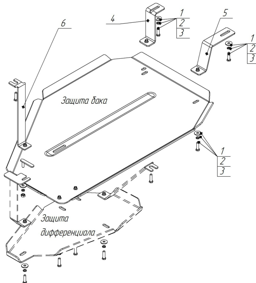
Схема установки
