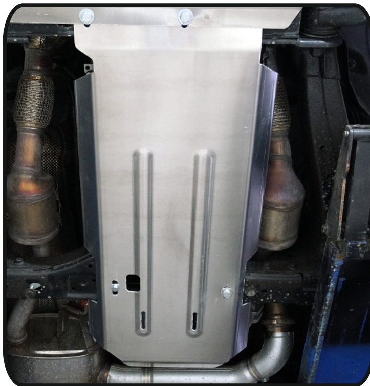
Защита КПП и раздаточной коробки (алюминий) 4мм арт.ZKTCC00624.
