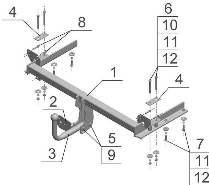
Рис.1. Схема сборки ТСУ.
