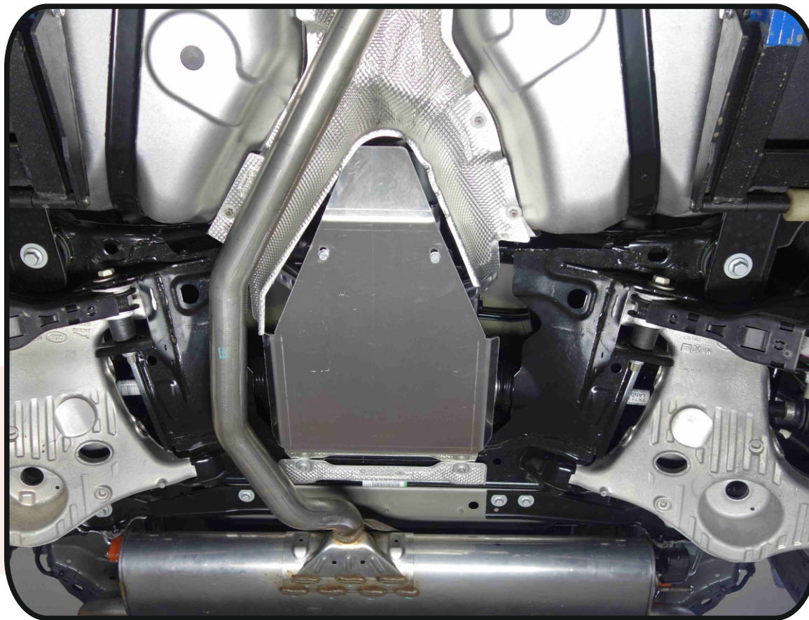
Защита дифференциала (алюминий) 4 мм арт. ZKTCC00186
