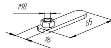
Закладной кронштейн z-47
