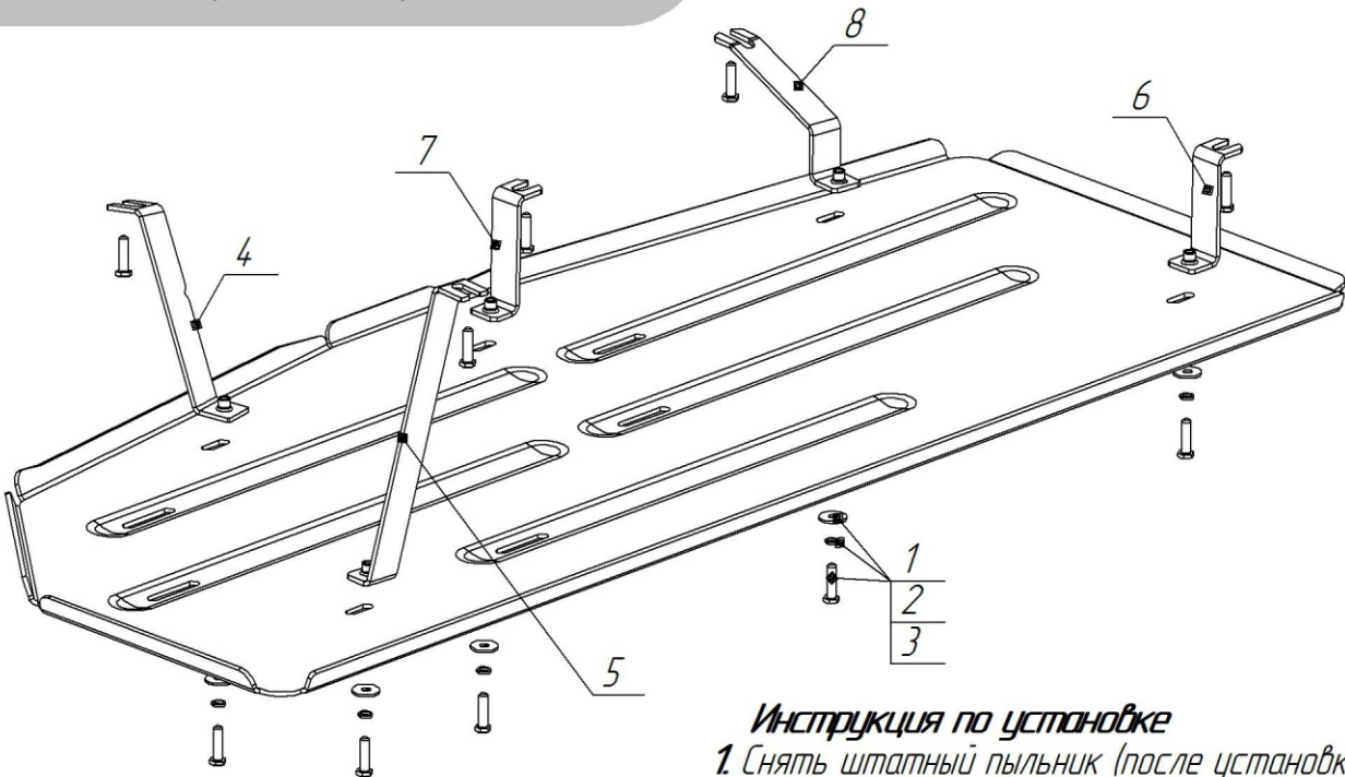
Схема установки
