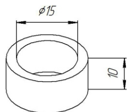
Втулка L=10 мм (поз.7)
