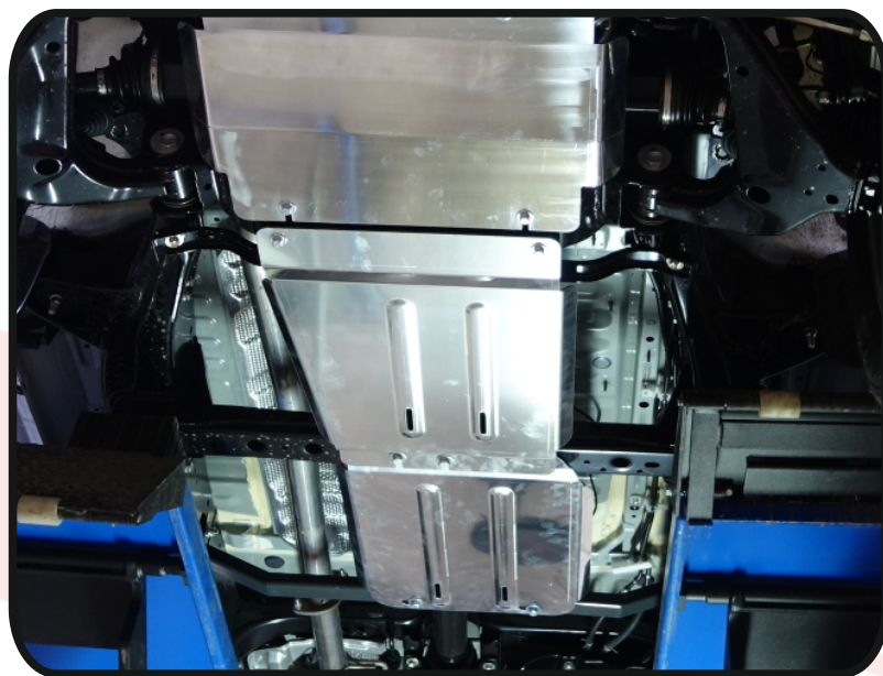
Защита КПП (алюминий) 4 мм арт. ZKTCC00031
