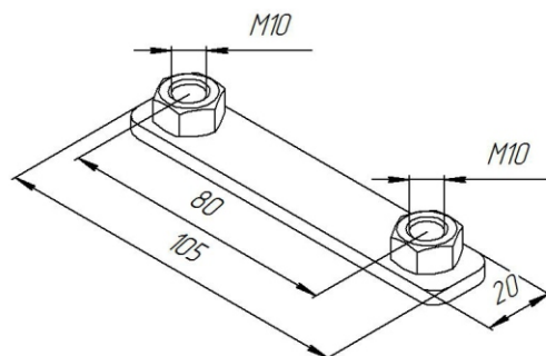
Закладной кронштейн (поз.8)
