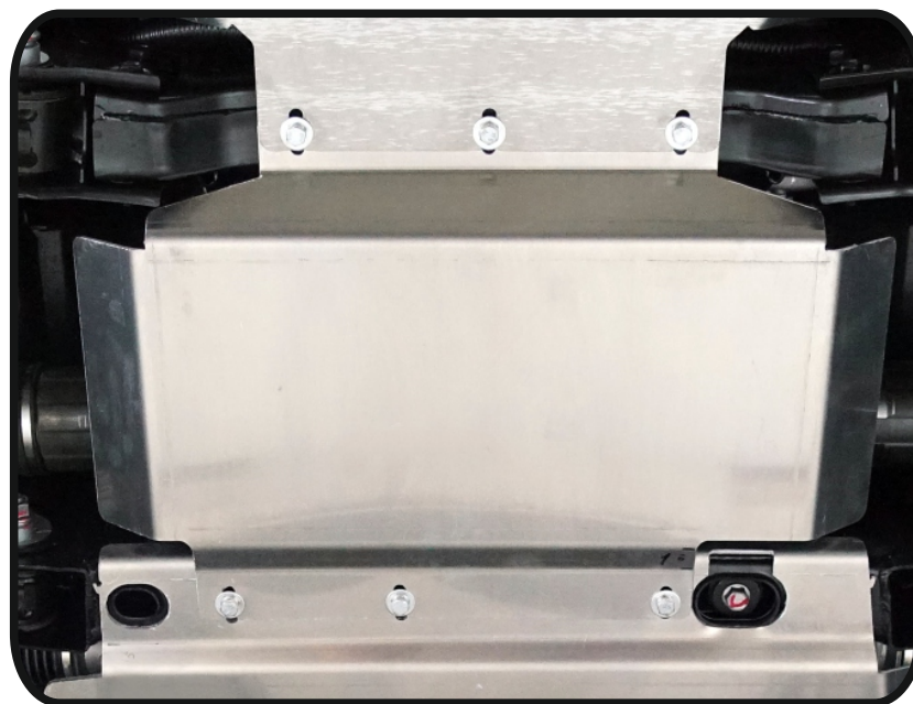
Защита картера и переднего редуктора(алюминий) 4 мм арт.ZKTCC00463.
