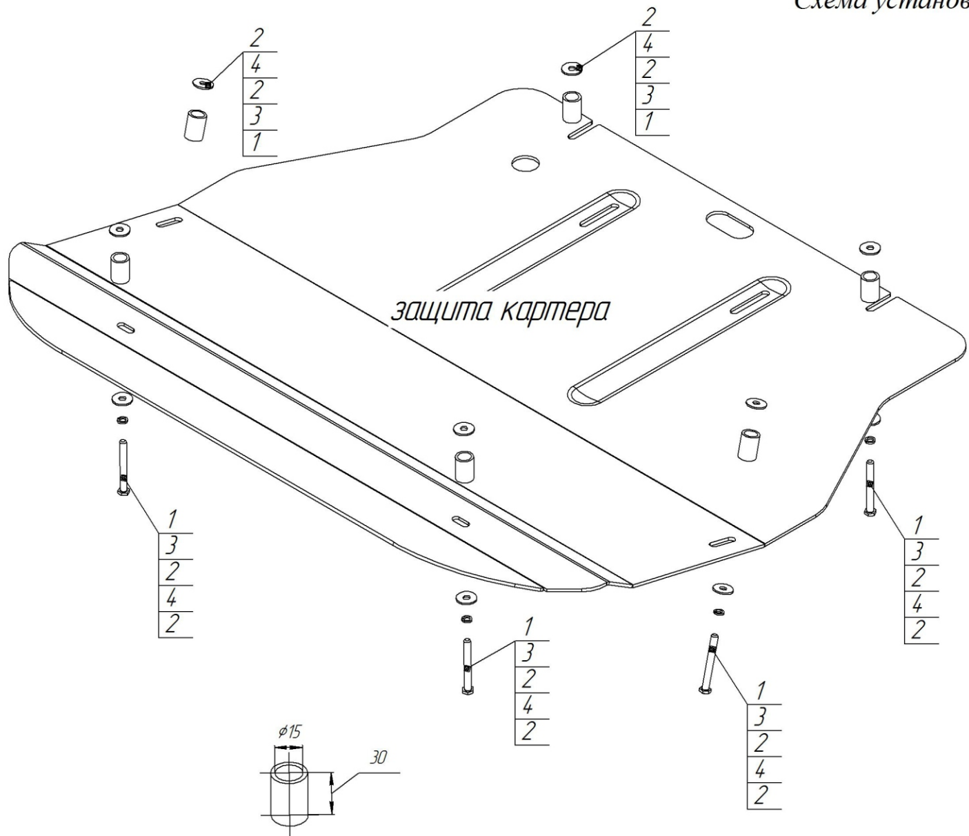
Втулка (поз.4)
