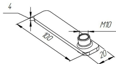
Закладной кронштейн M10 100x20
