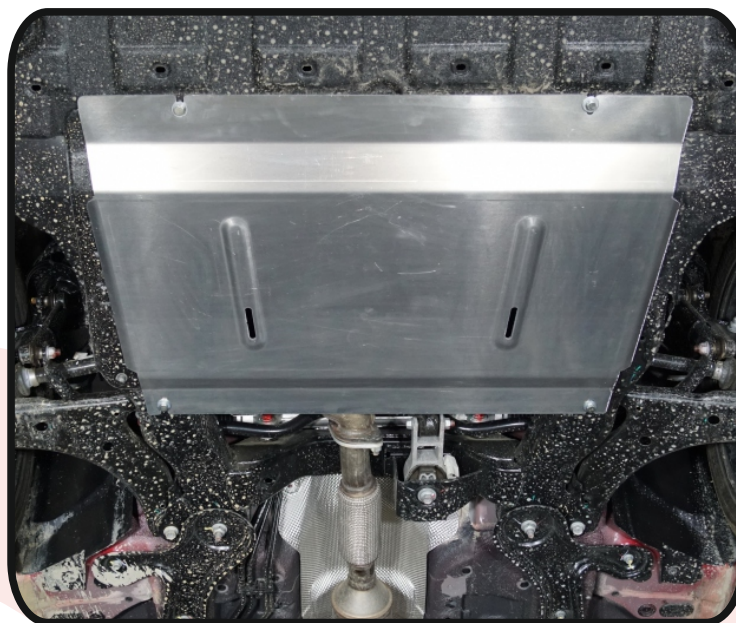
Защита картера и КПП (алюминий) 4 мм арт. ZKTCC00545.
