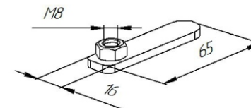
Закладной кронштейн Z47
